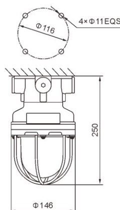
X: 吸顶式 Ceiling type
