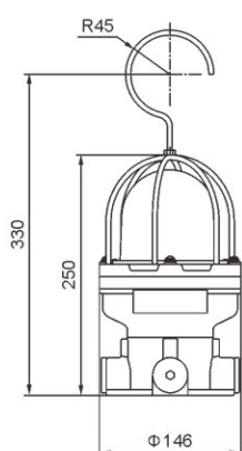
H: 手提式 Portable type
