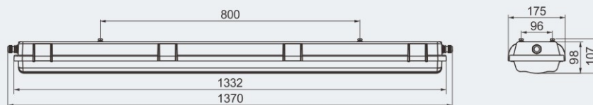
Type II: BnY81-LED 28 x 2□, BnY81-LED 28 x 2□J; BnY81-LED 40□J, BnY81-LED 60□, BnY81-LED 60□J
